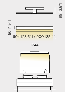
APPLICATION EXAMPLE ESEMPIO APPLICAZIONE
