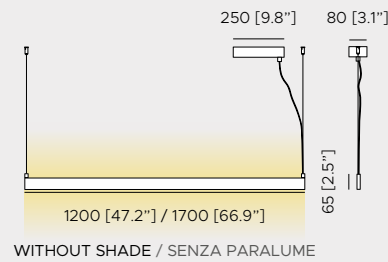
WITHOUT SHADE / SENZA PARALUME
